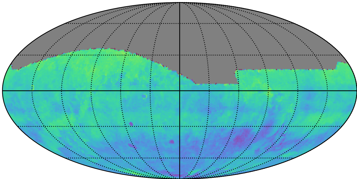
weather_cloudso2v3.4_10yrs i: Kuiper rotSkyPos
