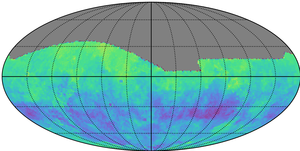
weather_cloudso2v3.4_10yrs g: Kuiper rotSkyPos
