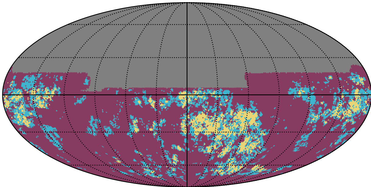
weather_cloudso2v3.4_10yrs y band: Gaps_7hr
