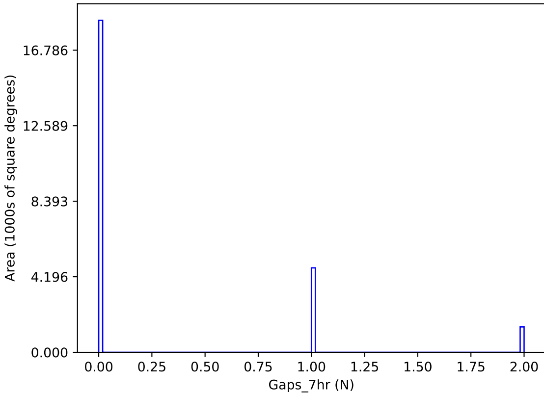
weather_cloudso2v3.4_10yrs y band: Gaps_7hr
