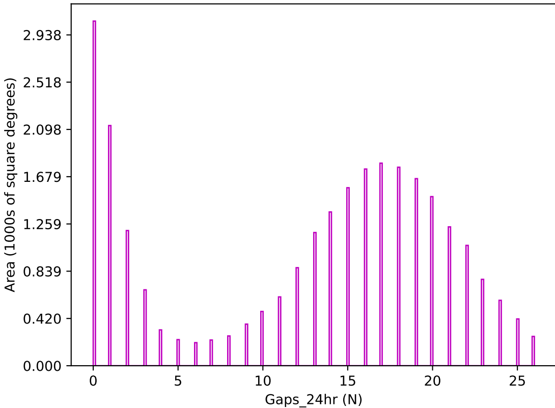
weather_cloudso2v3.4_10yrs z band: Gaps_24hr
