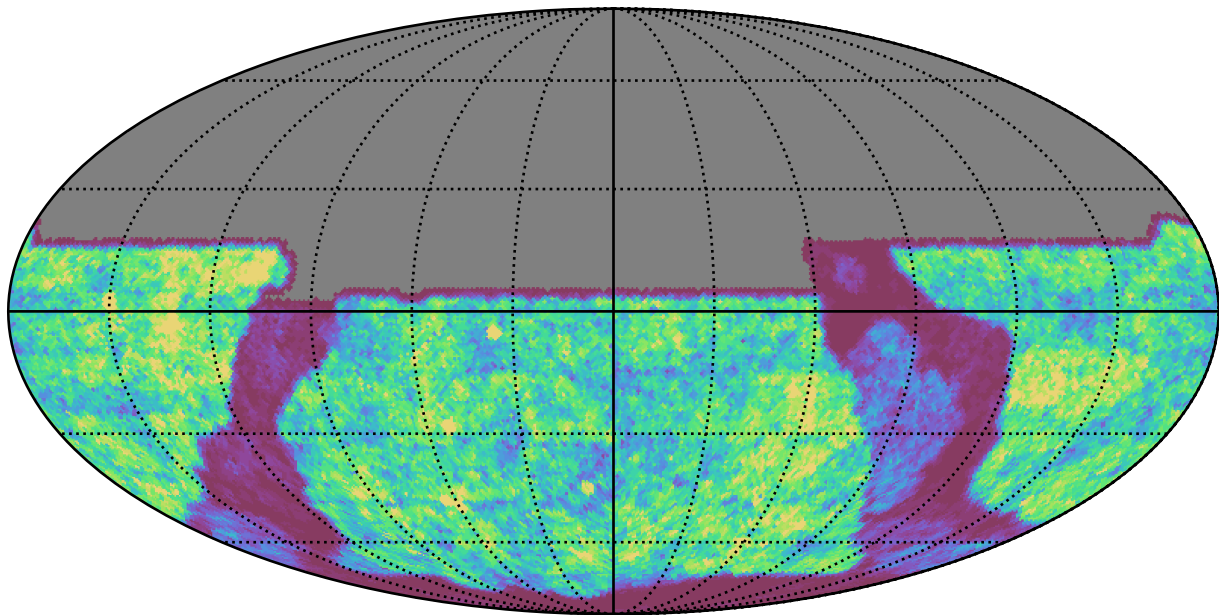
weather_cloudso2v3.4_10yrs y band: Gaps_24hr
