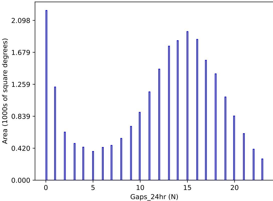
weather_cloudso2v3.4_10yrs y band: Gaps_24hr
