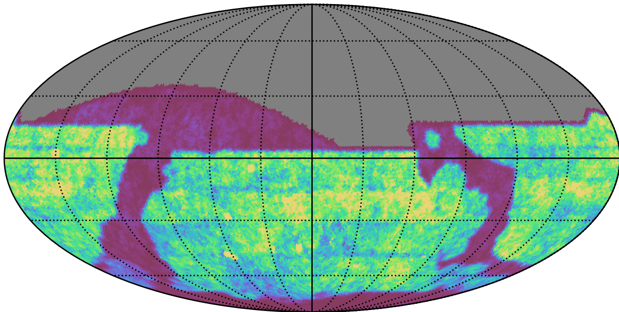
weather_cloudso2v3.4_10yrs r band: Gaps_24hr
