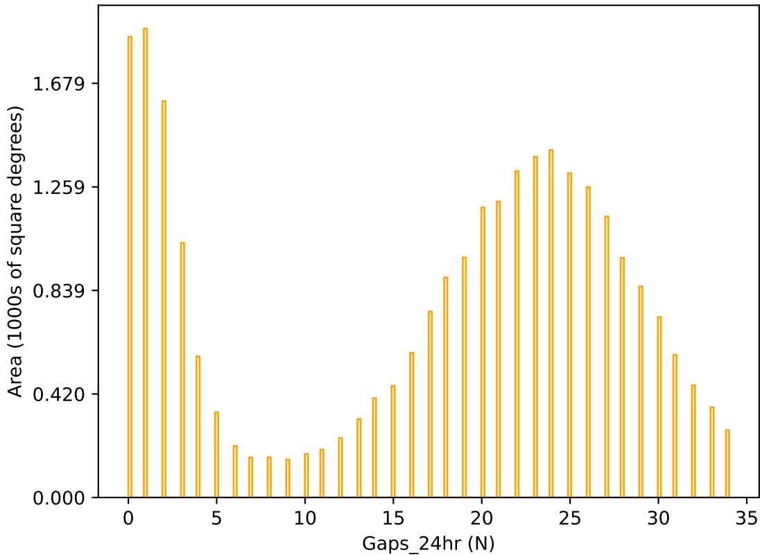
weather_cloudso2v3.4_10yrs r band: Gaps_24hr
