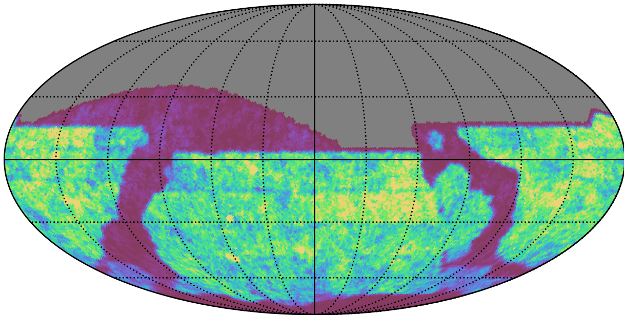
weather_cloudso2v3.4_10yrs i band: Gaps_24hr
