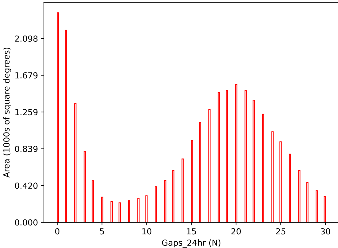
weather_cloudso2v3.4_10yrs i band: Gaps_24hr
