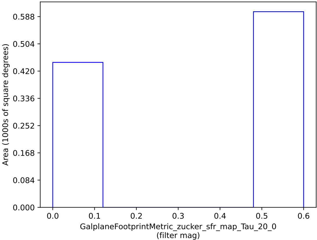
weather_cloudso2v3.4_10yrs : GalplaneFootprintMetric_zucker_sfr_map_Tau_20_0
