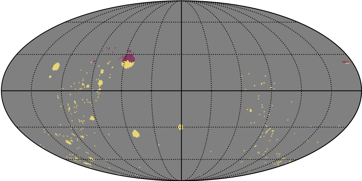
weather_cloudso2v3.4_10yrs : GalplaneFootprintMetric_open_clusters_map_Tau_46_5
