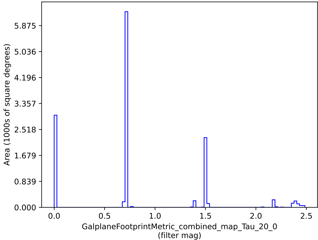
weather_cloudso2v3.4_10yrs : GalplaneFootprintMetric_combined_map_Tau_20_0
