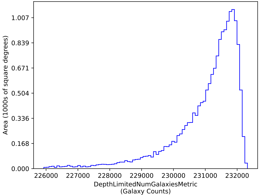
weather_cloudso2v3.4_10yrs i band galaxies non-DD: DepthLimitedNumGalaxiesMetric
