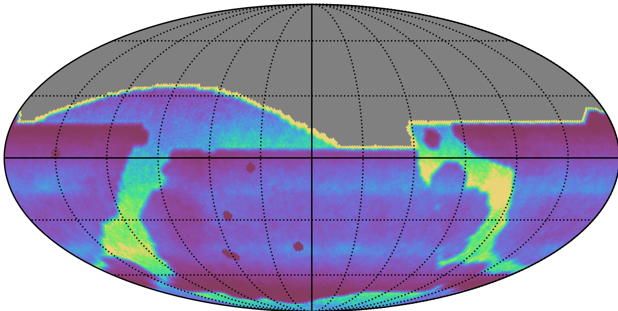
weather_cloudso2v3.4_10yrs : DCRprecision
