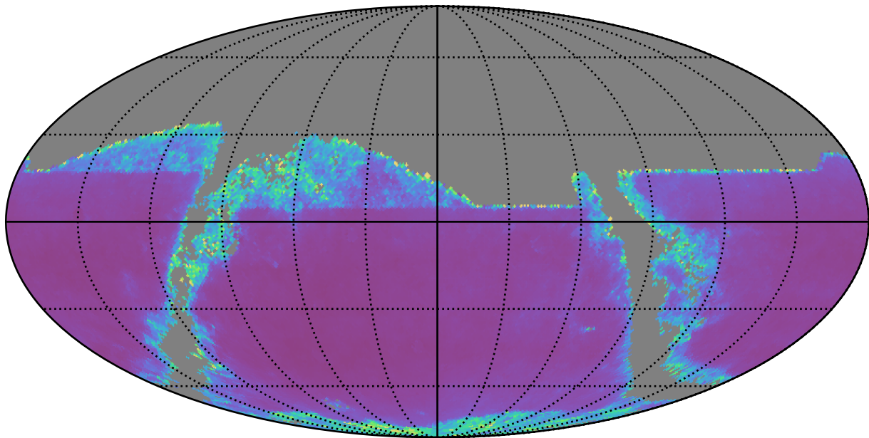
weather_cloudso2v3.4_10yrs z band: AGN SF_uncert
