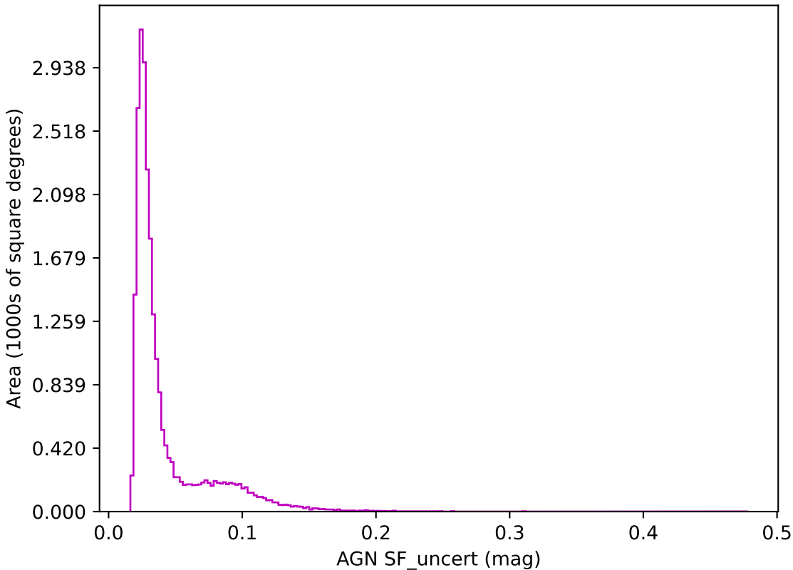
weather_cloudso2v3.4_10yrs z band: AGN SF_uncert
