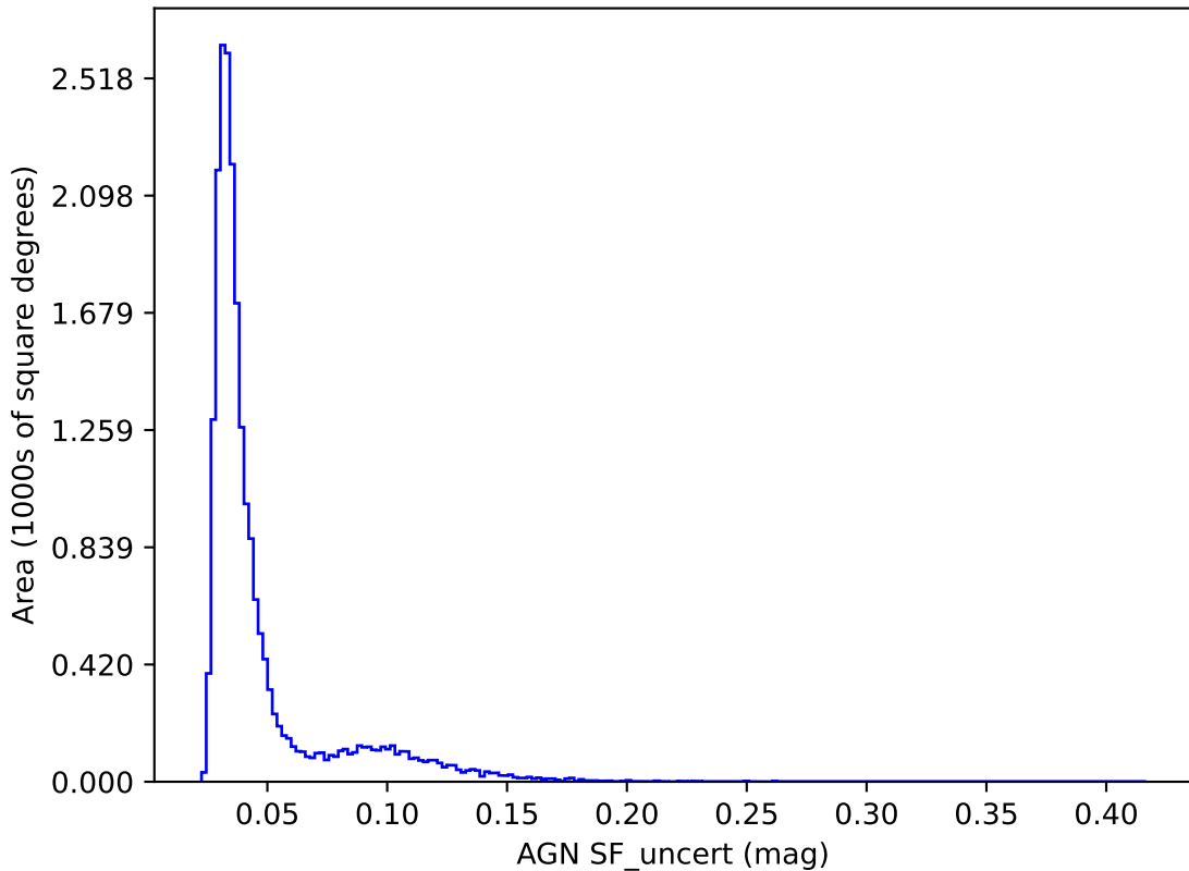
weather_cloudso2v3.4_10yrs y band: AGN SF_uncert
