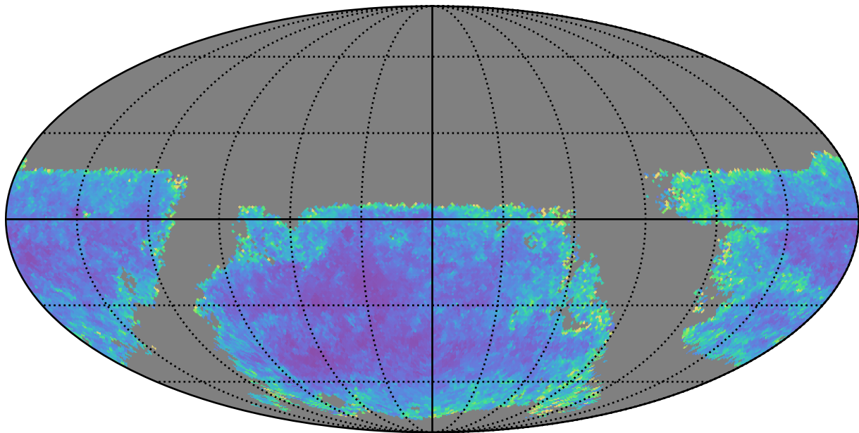
weather_cloudso2v3.4_10yrs u band: AGN SF_uncert
