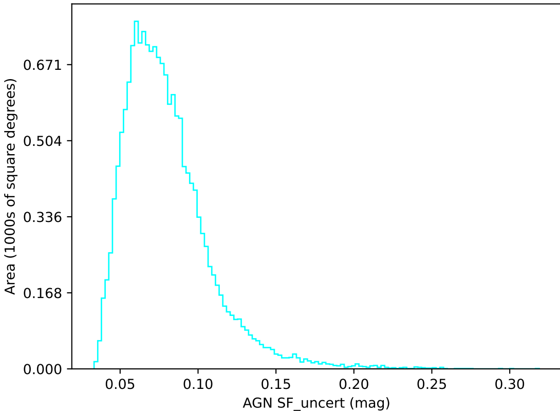
weather_cloudso2v3.4_10yrs u band: AGN SF_uncert
