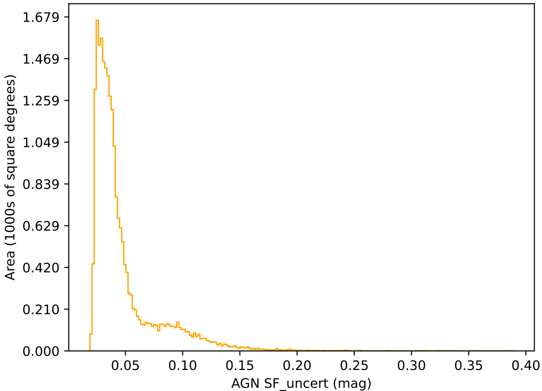
weather_cloudso2v3.4_10yrs r band: AGN SF_uncert
