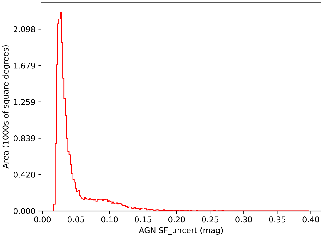
weather_cloudso2v3.4_10yrs i band: AGN SF_uncert
