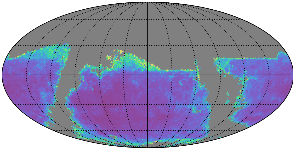
weather_cloudso2v3.4_10yrs g band: AGN SF_uncert
