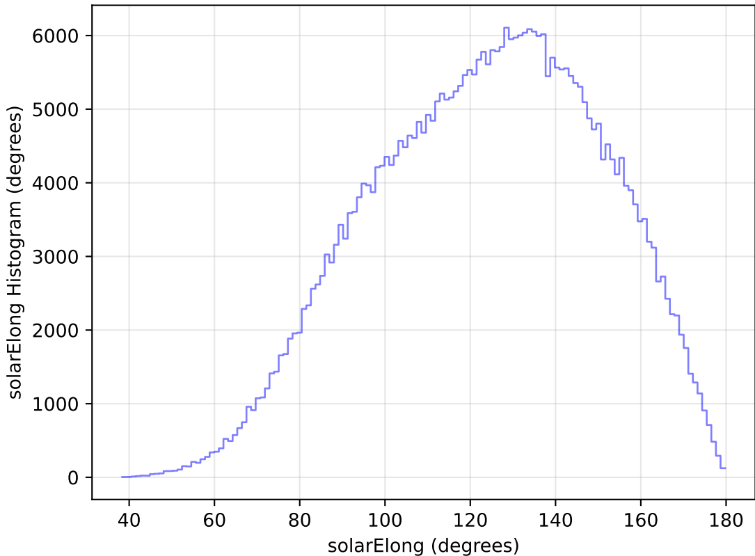
weather_cloudso2v3.4_10yrs WFD y band: solarElong Histogram
