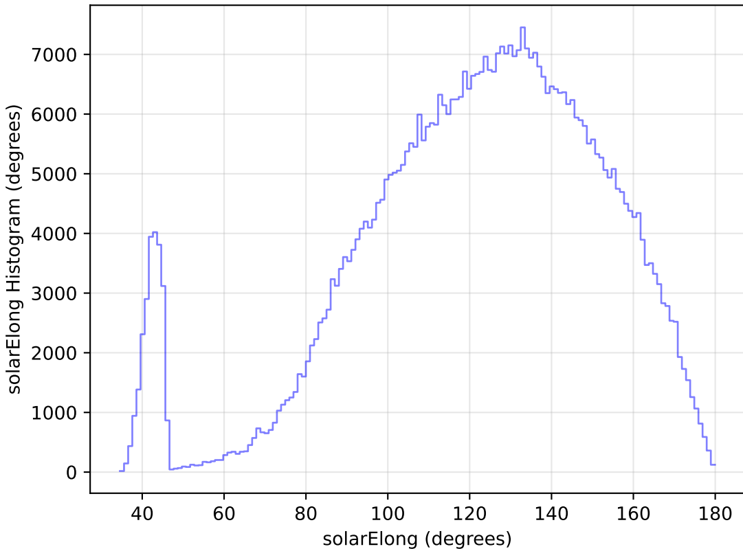
weather_cloudso2v3.4_10yrs WFD i band: solarElong Histogram
