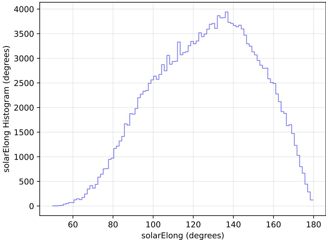
weather_cloudso2v3.4_10yrs WFD g band: solarElong Histogram
