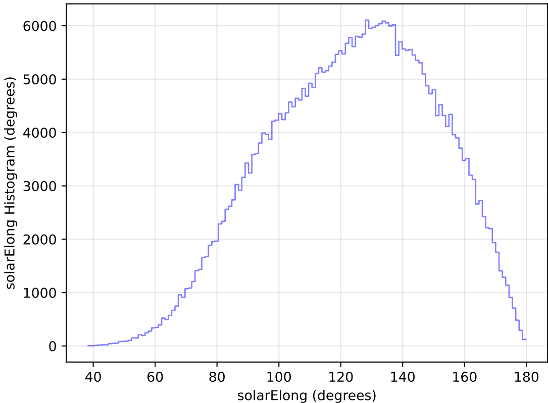
weather_cloudso2v3.4_10yrs All sky y band: solarElong Histogram
