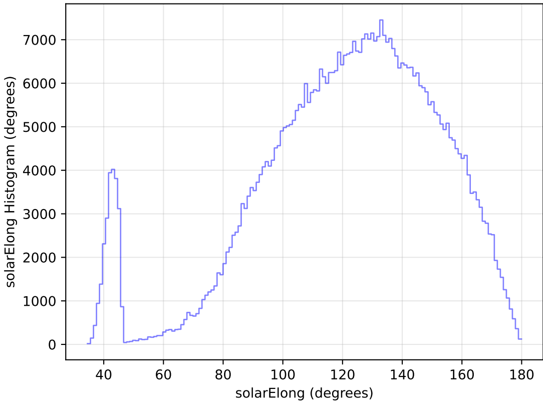
weather_cloudso2v3.4_10yrs All sky i band: solarElong Histogram
