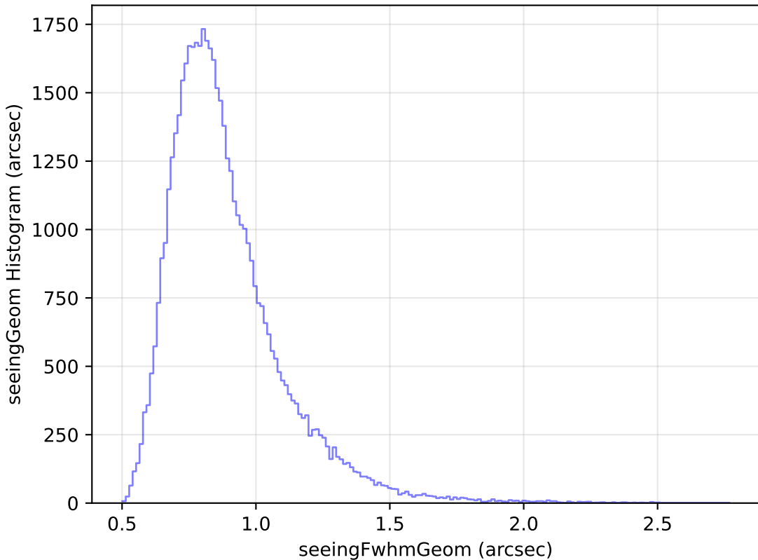
weather_cloudso2v3.4_10yrs Yr 1 y band: seeingGeom Histogram
