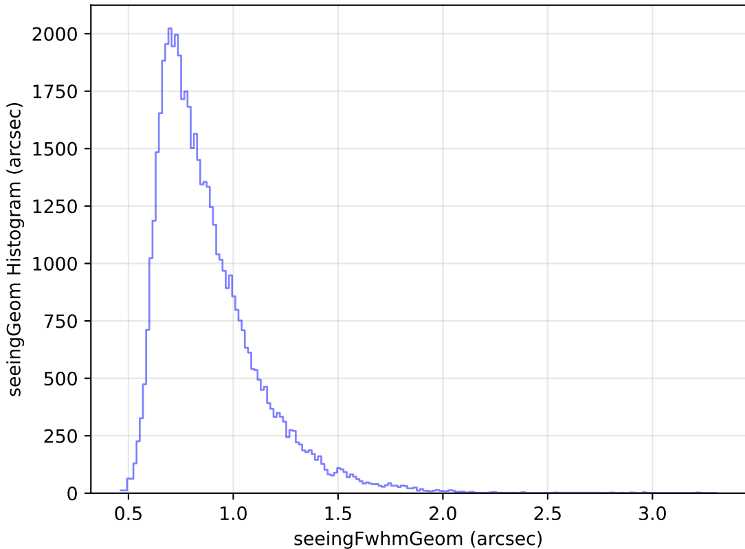
weather_cloudso2v3.4_10yrs Yr 1 r band: seeingGeom Histogram
