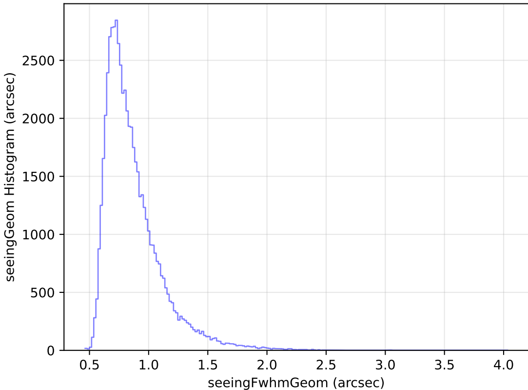
weather_cloudso2v3.4_10yrs Yr 1 i band: seeingGeom Histogram
