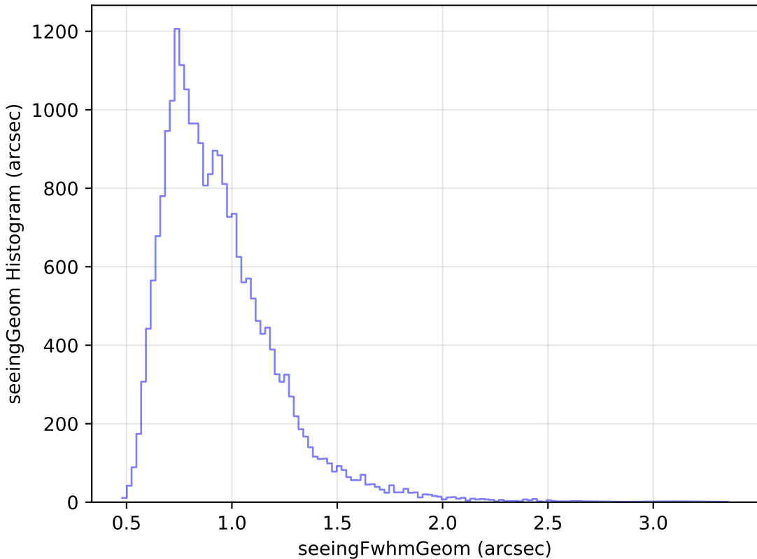
weather_cloudso2v3.4_10yrs Yr 1 g band: seeingGeom Histogram
