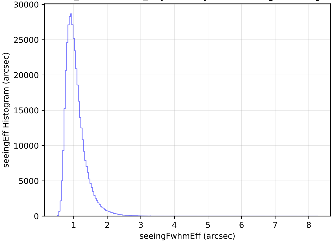
weather_cloudso2v3.4_10yrs WFD y band: seeingEff Histogram
