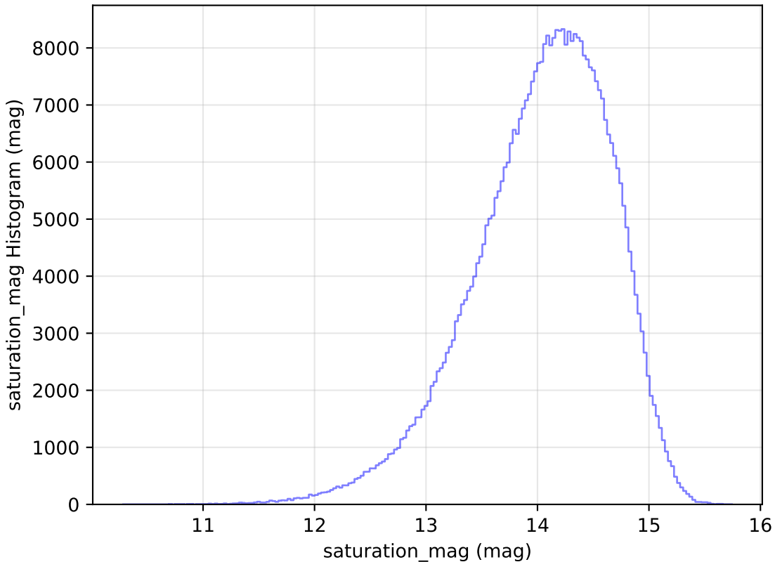
weather_cloudso2v3.4_10yrs WFD z band: saturation_mag Histogram
