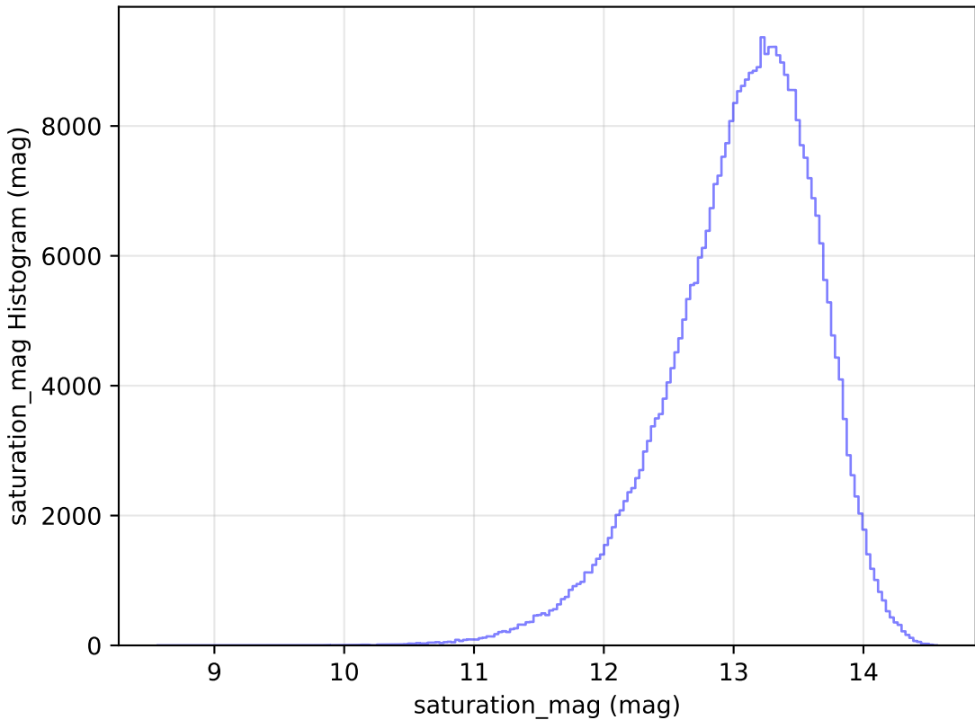
weather_cloudso2v3.4_10yrs WFD y band: saturation_mag Histogram
