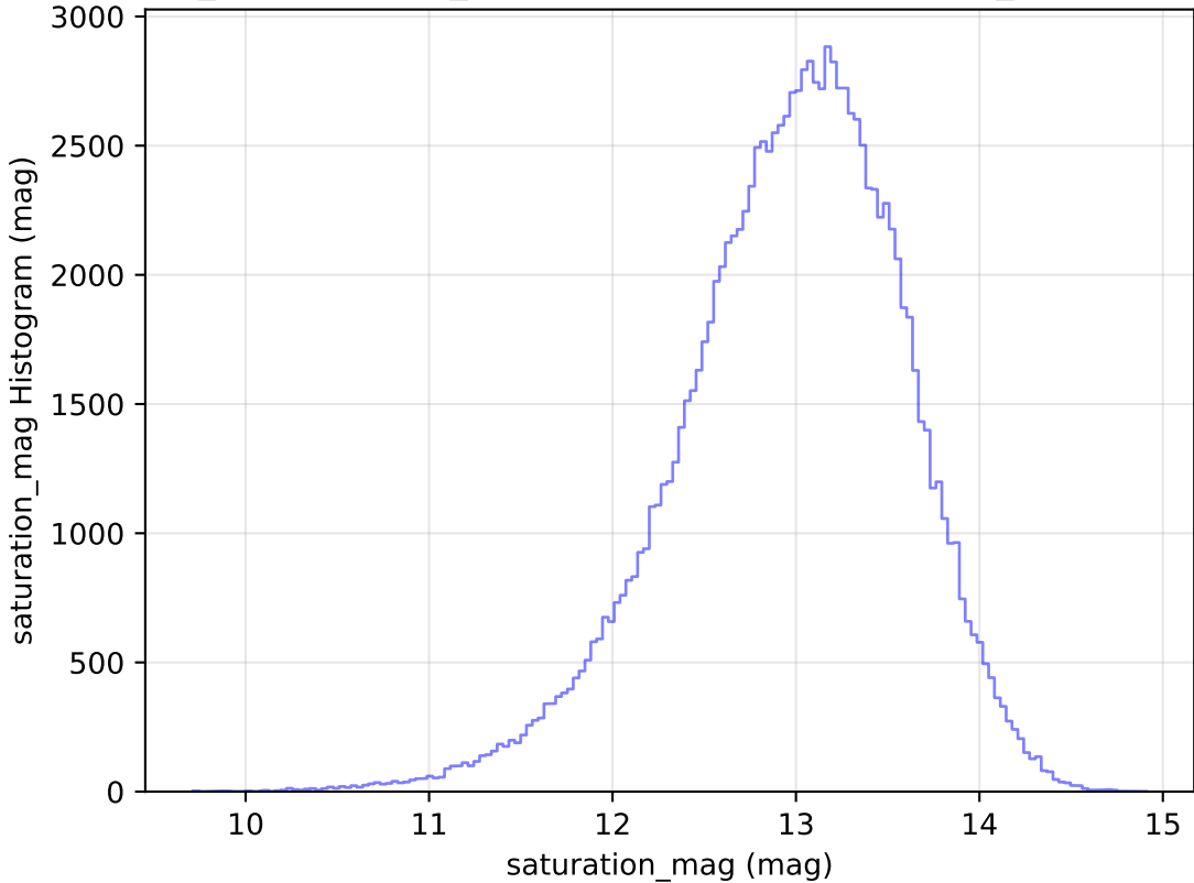
weather_cloudso2v3.4_10yrs WFD u band: saturation_mag Histogram
