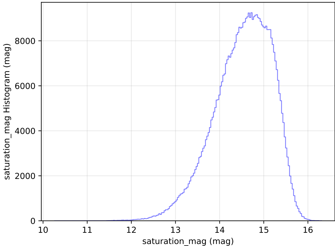
weather_cloudso2v3.4_10yrs WFD r band: saturation_mag Histogram
