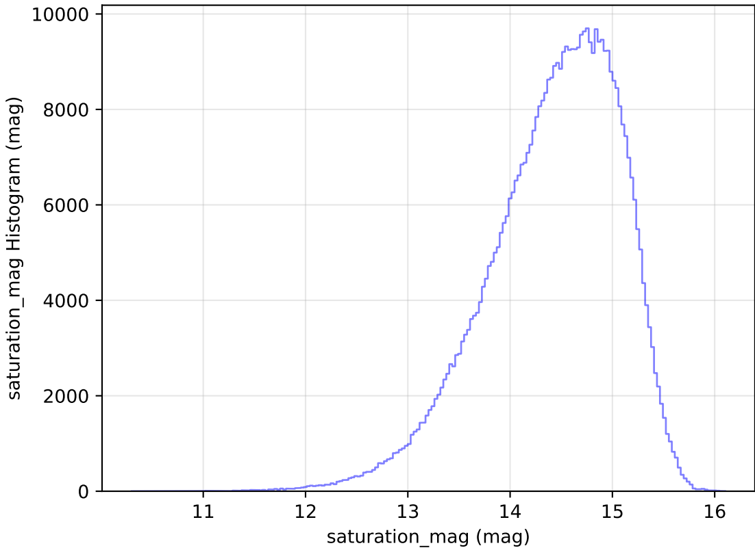
weather_cloudso2v3.4_10yrs WFD i band: saturation_mag Histogram
