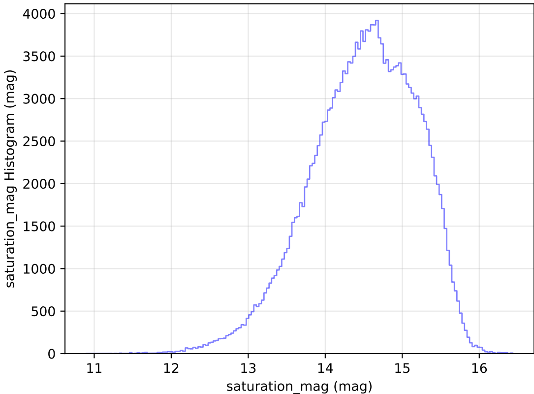
weather_cloudso2v3.4_10yrs WFD g band: saturation_mag Histogram
