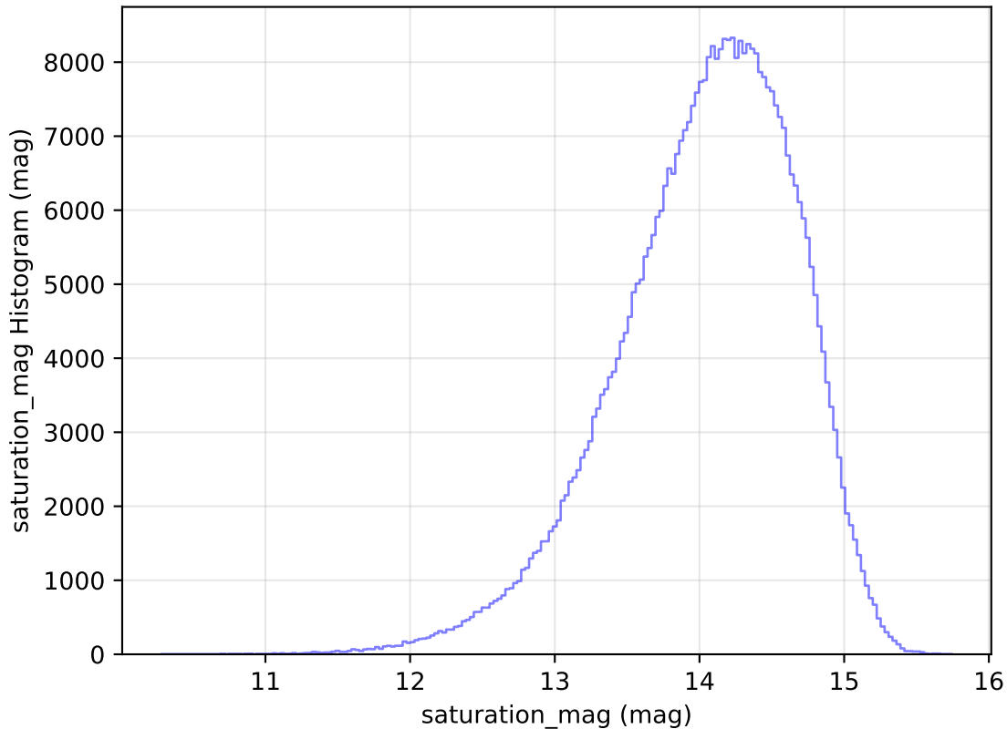
weather_cloudso2v3.4_10yrs All sky z band: saturation_mag Histogram
