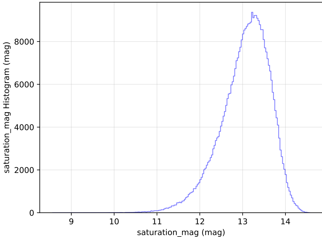
weather_cloudso2v3.4_10yrs All sky y band: saturation_mag Histogram
