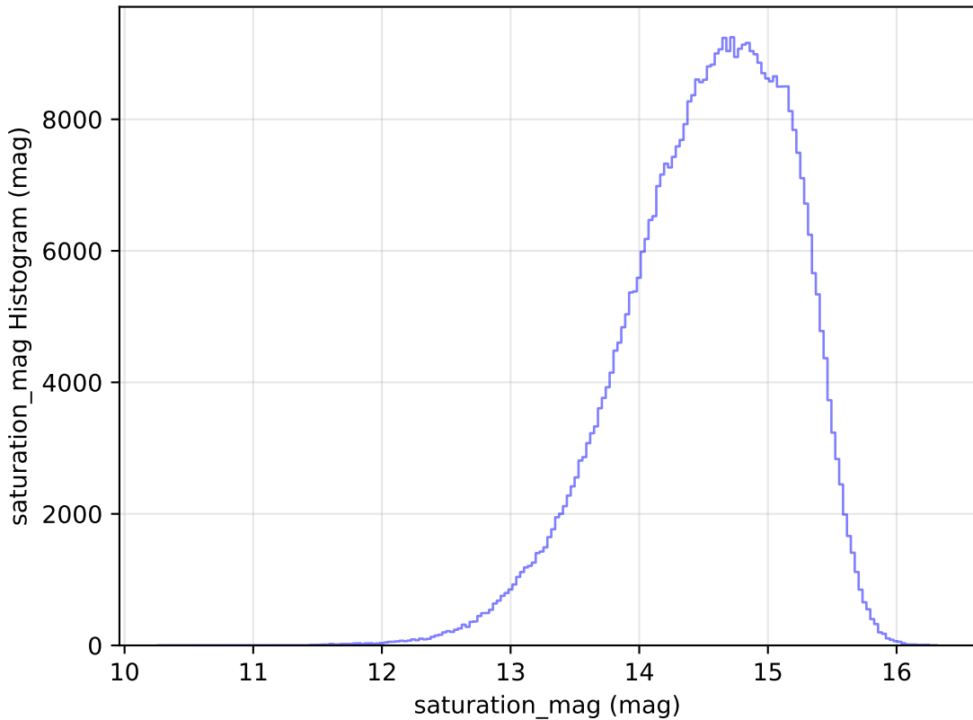
weather_cloudso2v3.4_10yrs All sky r band: saturation_mag Histogram
