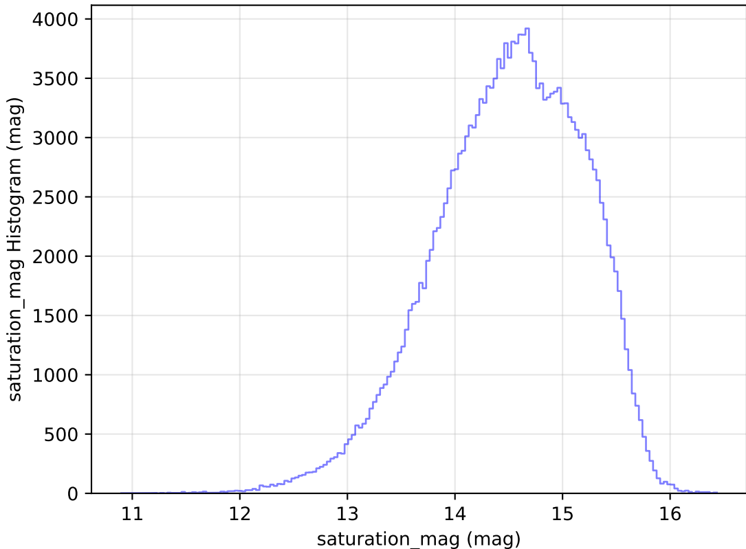
weather_cloudso2v3.4_10yrs All sky g band: saturation_mag Histogram
