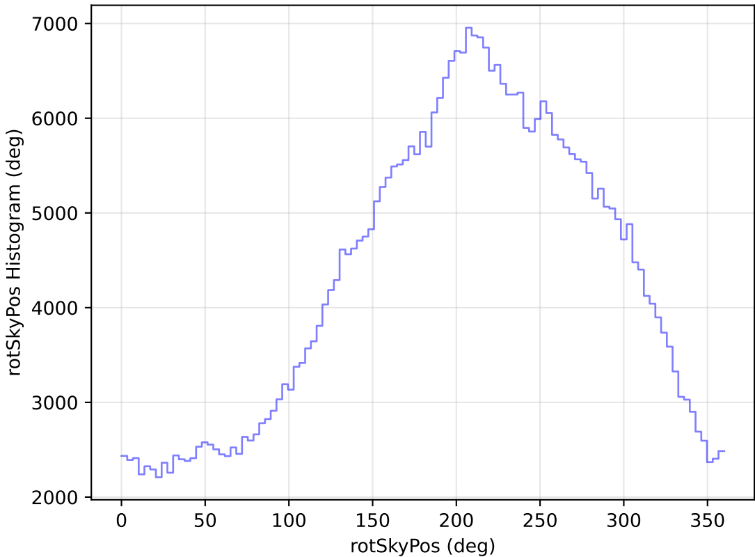
weather_cloudso2v3.4_10yrs WFD z band: rotSkyPos Histogram
