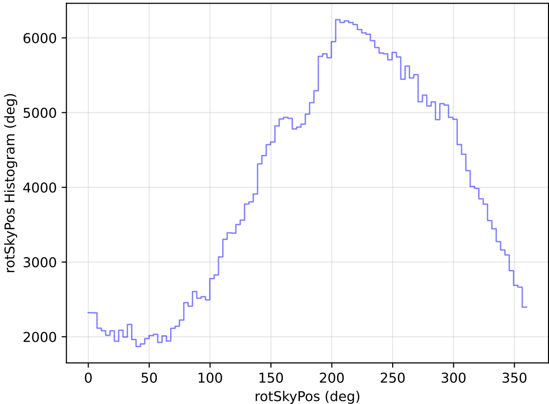
weather_cloudso2v3.4_10yrs WFD y band: rotSkyPos Histogram
