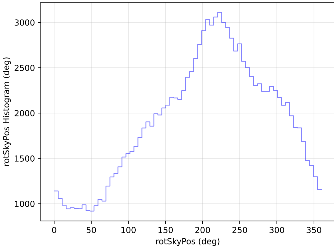
weather_cloudso2v3.4_10yrs WFD u band: rotSkyPos Histogram
