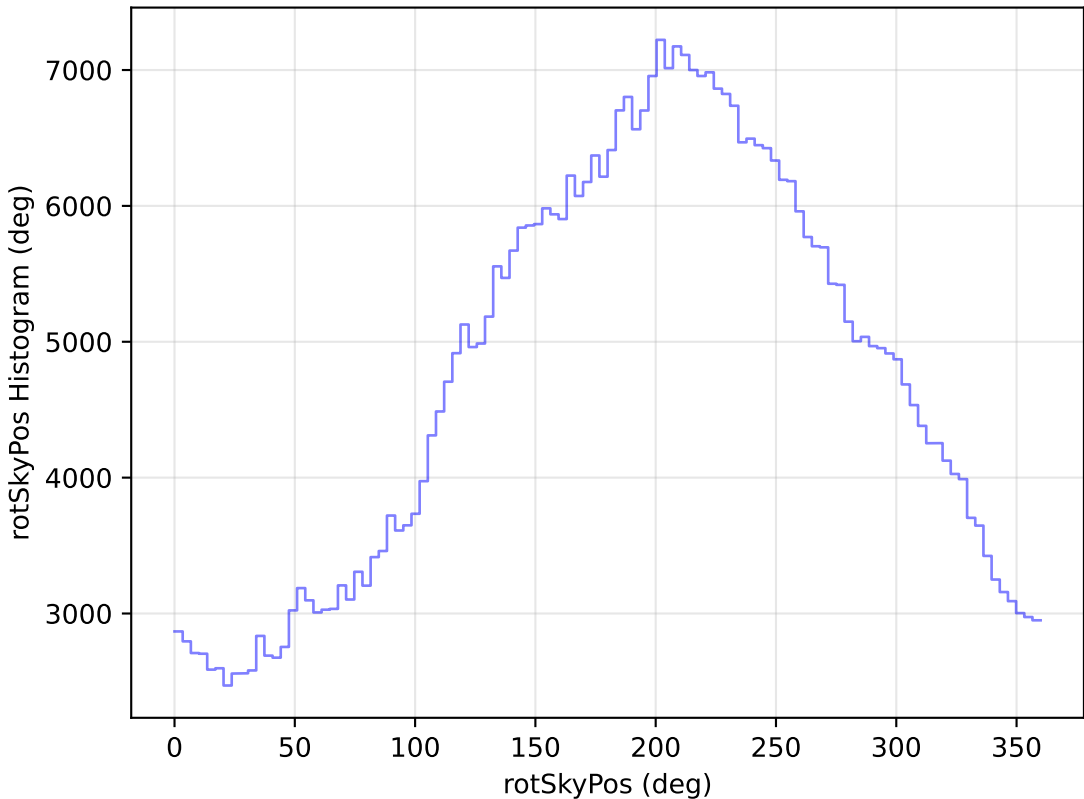
weather_cloudso2v3.4_10yrs WFD r band: rotSkyPos Histogram
