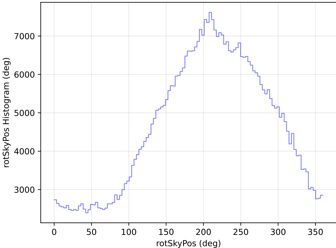
weather_cloudso2v3.4_10yrs WFD i band: rotSkyPos Histogram
