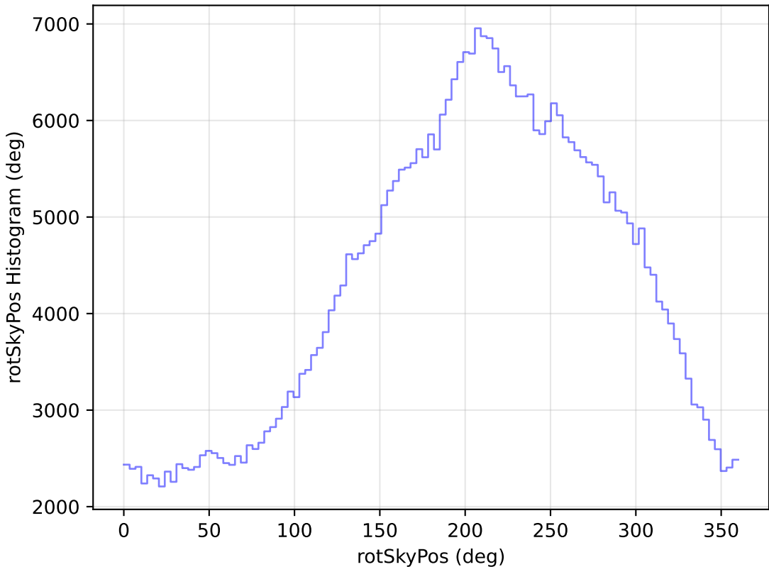
weather_cloudso2v3.4_10yrs All sky z band: rotSkyPos Histogram
